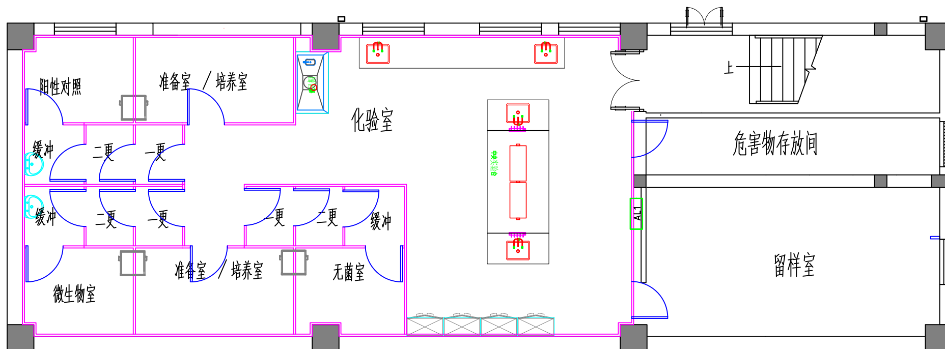
化验室布置图
